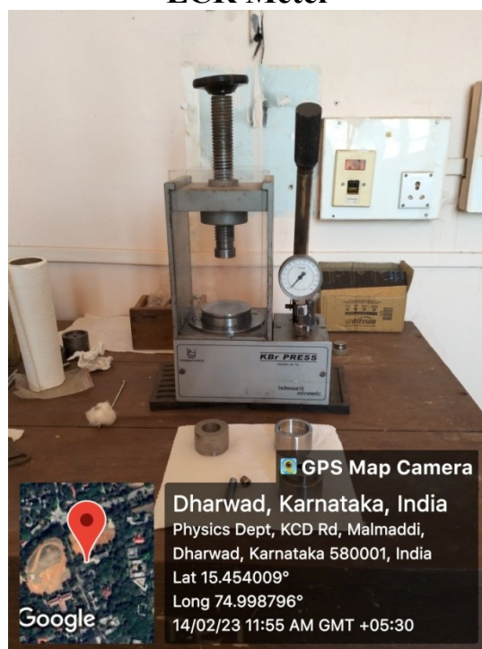
KBr Press
