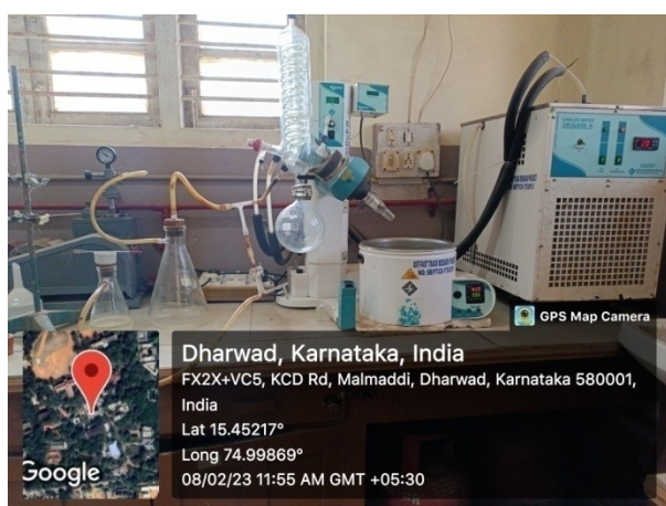
Rota Evaporator
